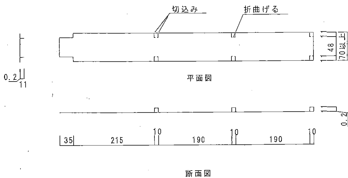
耐熱シール材充てん用鋼板円筒展開図
