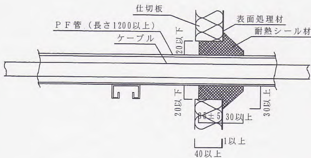
D-D' 断面図
