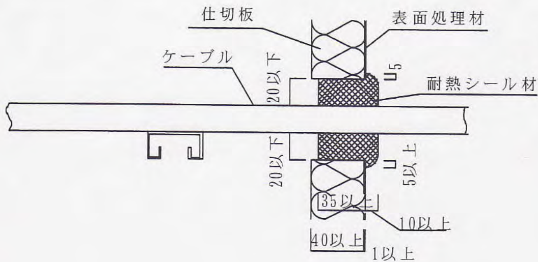
E-E' 断面図
