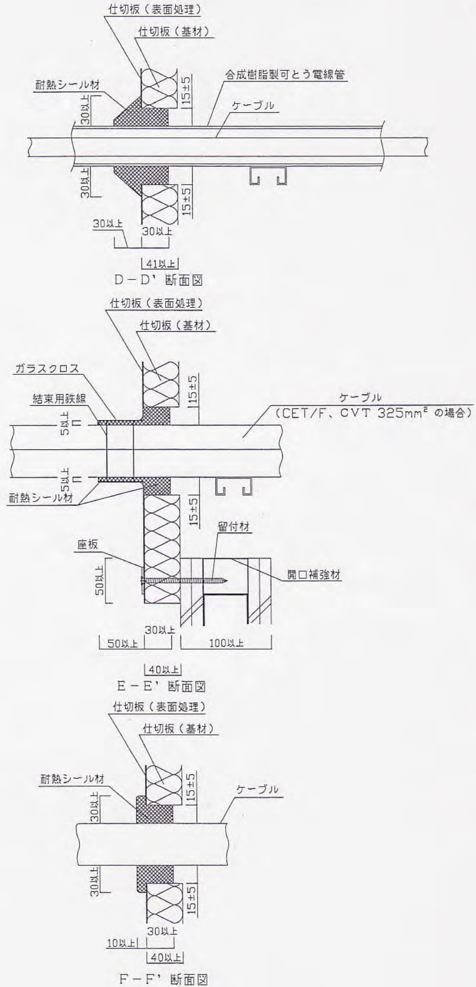
図3 構造説明図
