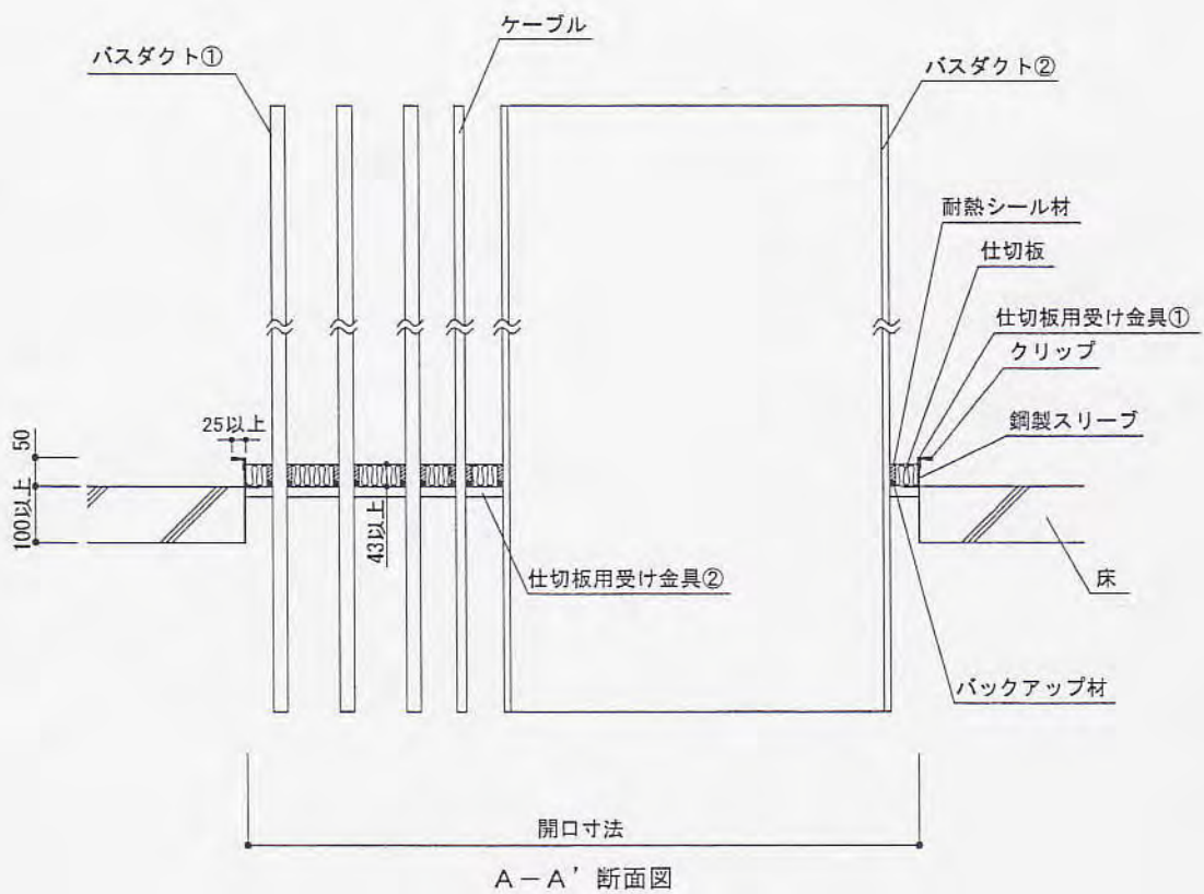
図1 構造説明図
