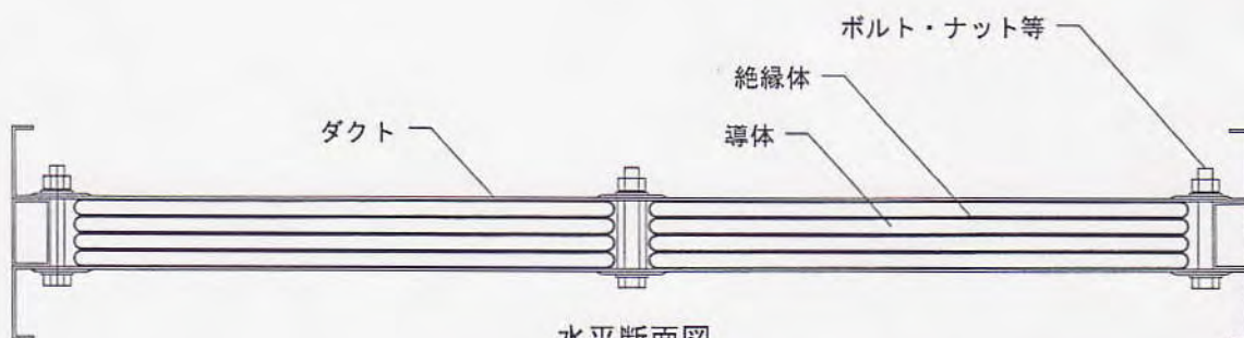
水平断面図
