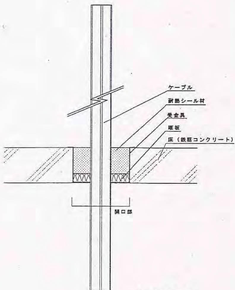
A-A' 断面図
