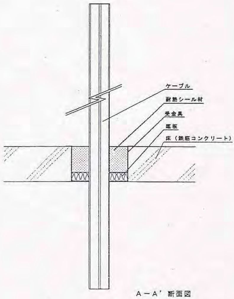
図3 施工図
