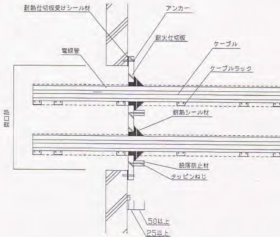
C-C' 断面図
